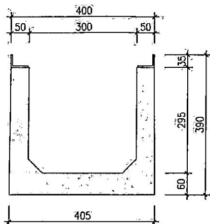
SEZIONE A-A
